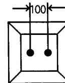
12 m φ 台形塚石 (アンカーボルト付) 170/260×600
